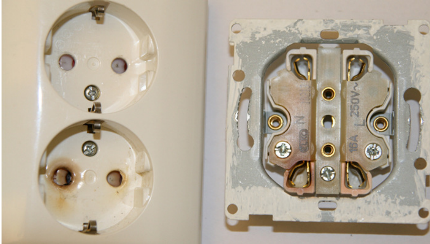
Skade/varmgang på kontakt ved manglende avlastning. (Foto: DSB)
